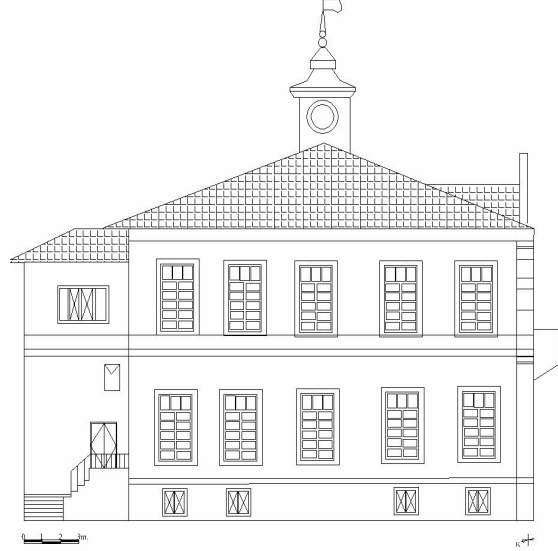
Çizim 4. Bergama Hükümet Konağı Güney Cephe
