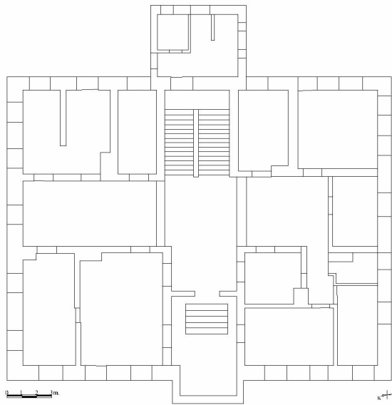
Plan 3. Bergama Hükümet Konağı Zemin Kat Planı
