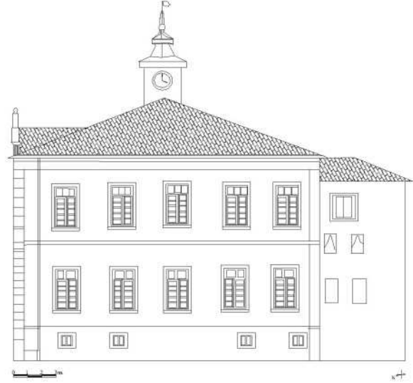
Çizim 3. Bergama Hükümet Konağı Kuzey Cephe
