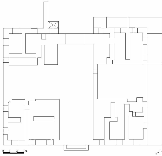
Plan 2. Bergama Hükümet Konağı Bodrum Kat Planı
