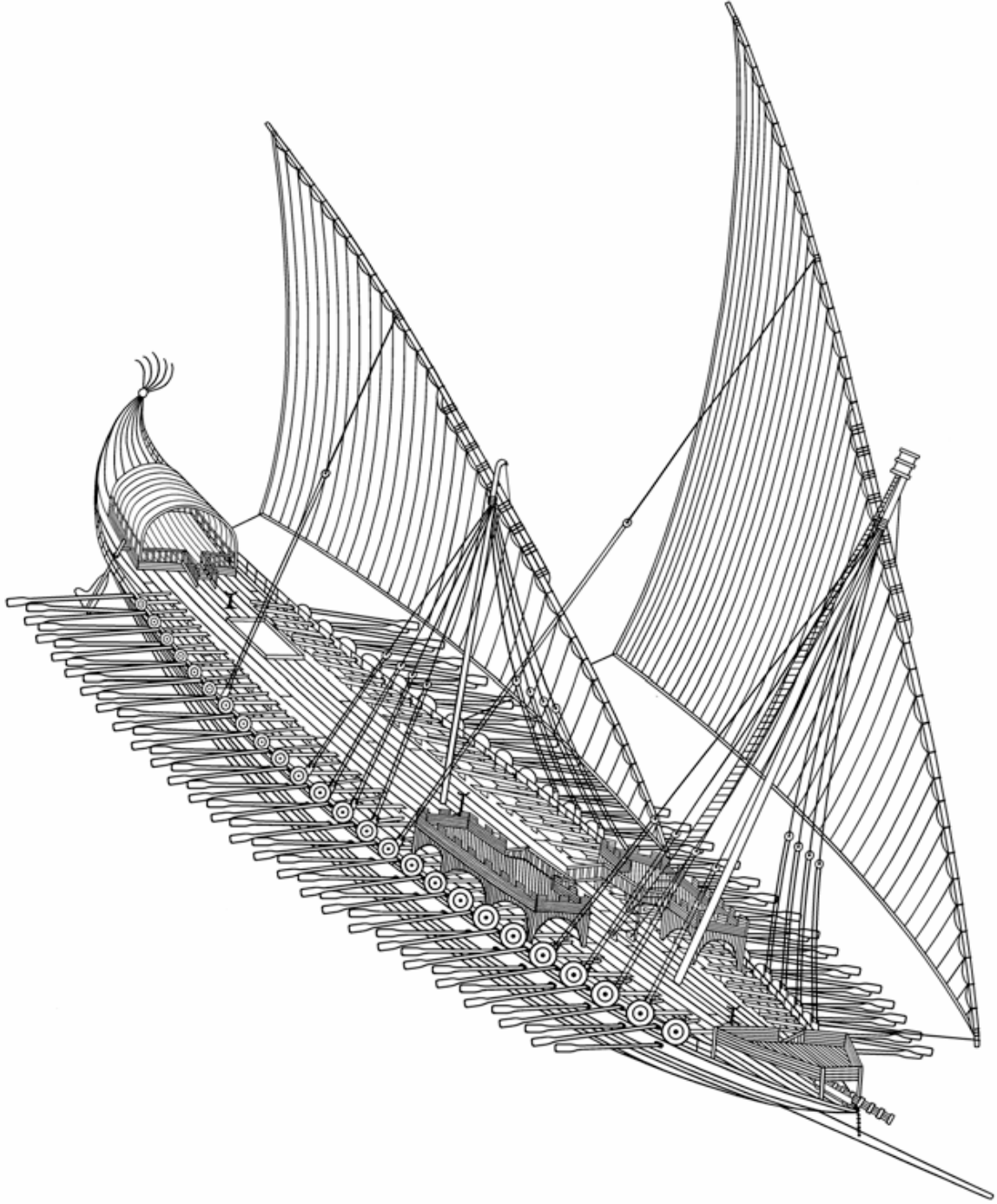
Fig.3: Bir dromonun rekonstrüksiyon çizimi(J.H.Proyor'dan)
