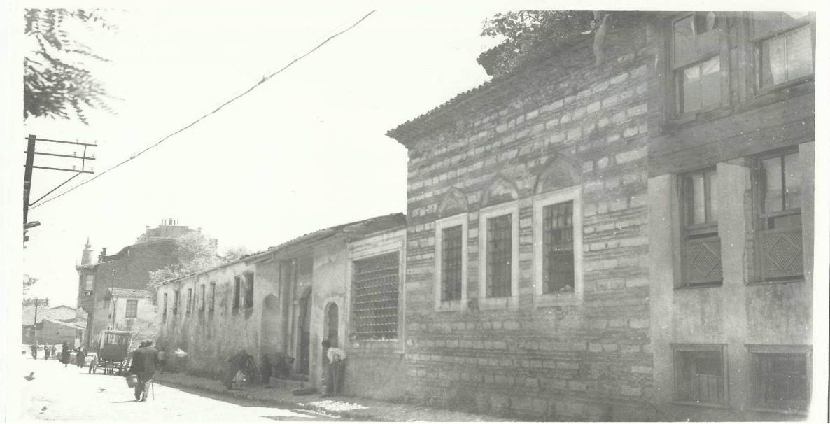
Kalenderhâne Tekkesi ve sıbyan mektebinin dıştan görünüşü, eski hâli (İstanbul Arkeoloji Müzesi Eski Eserler Encümen Arşivi, 1942, nr. 4925).
