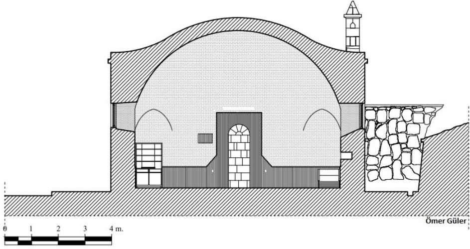
Çizim 3: Haydar Bey Camii En Kesiti (Ömer Güler'den)
