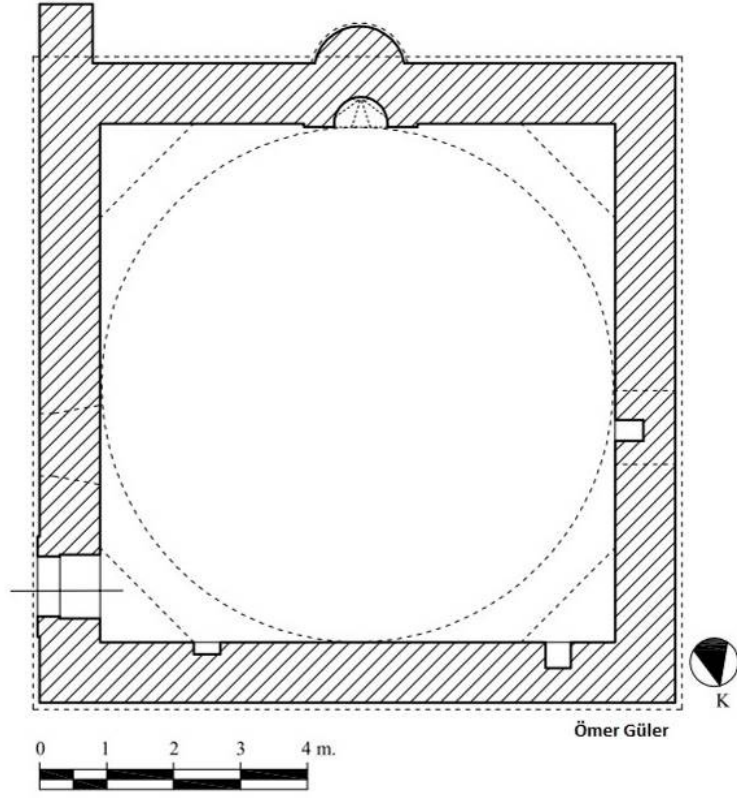
Çizim 1: Haydar Bey Camii Planı (Ömer Güler'den)
