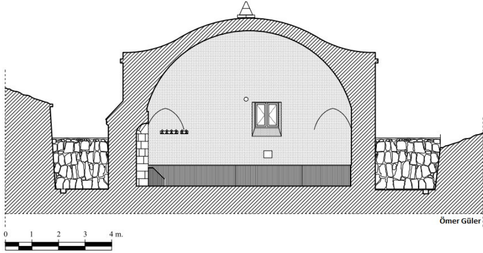
Çizim 2: Haydar Bey Camii Boy Kesiti (Ömer Güler'den)
