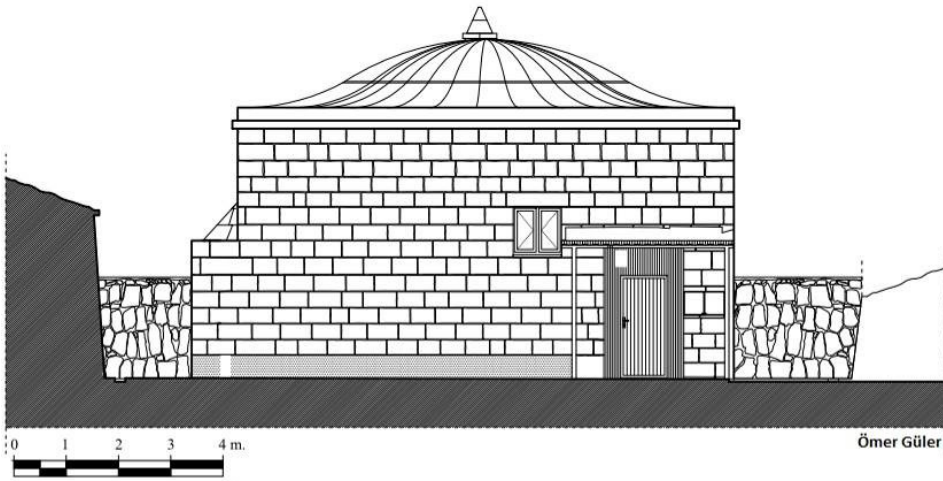
Çizim 5: Haydar Bey Camii Doğu Cephe Görünüşü (Ömer Güler'den)
