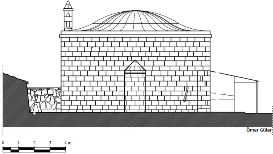
Çizim 4: Haydar Bey Camii Güney Cephe Görünüşü (Ömer Güler'den)
