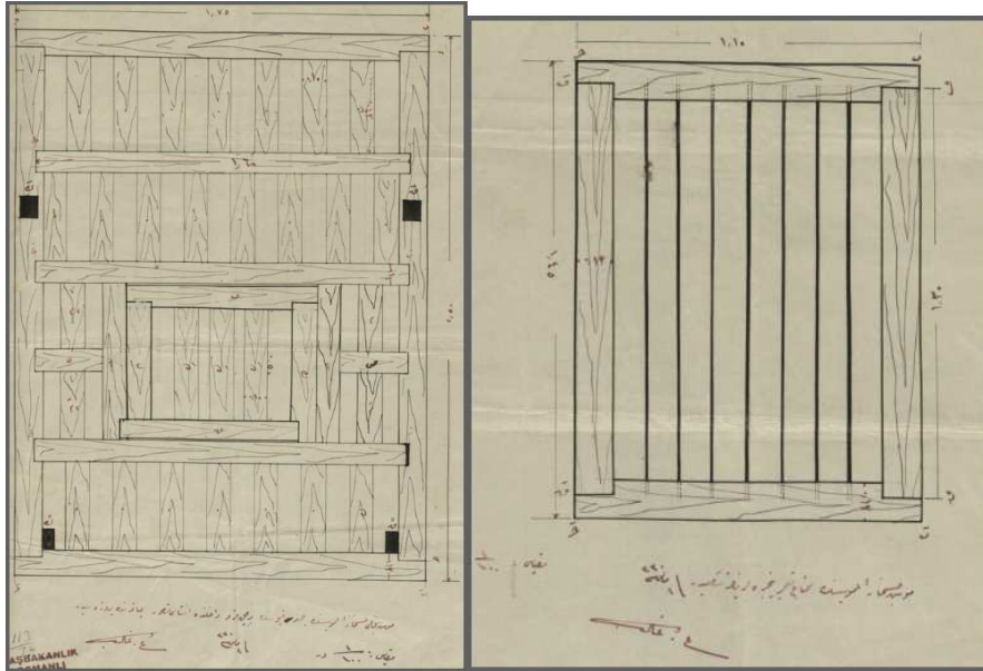
Şekil 2: Yapılması planlanan binanın yeni kapısı (solda) ve pencerelerini (sağda) gösteren taslak
