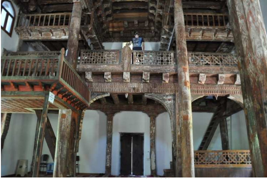
Şekil 18. Ahşap Kademeli Mahfil Sistemi
